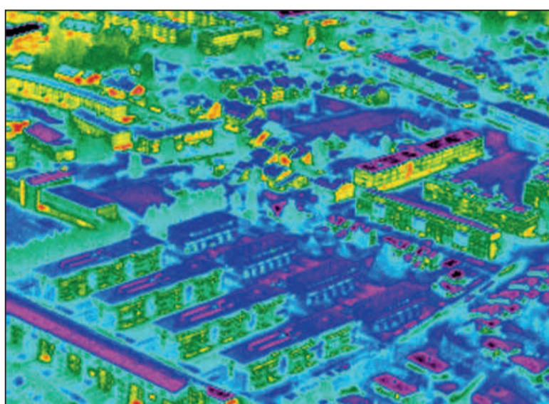
■ Image infrarouge du quartier Monthoux. Les immeubles MINERGIE situés au premier plan laissent apparaître des pertes de chaleur beaucoup plus faibles que les immeubles situés en arrière-plan.
