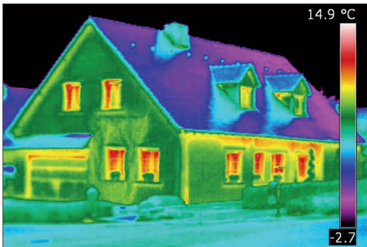
■ Mise en évidence des faiblesses de l'isolation lors d'une analyse par thermographie
