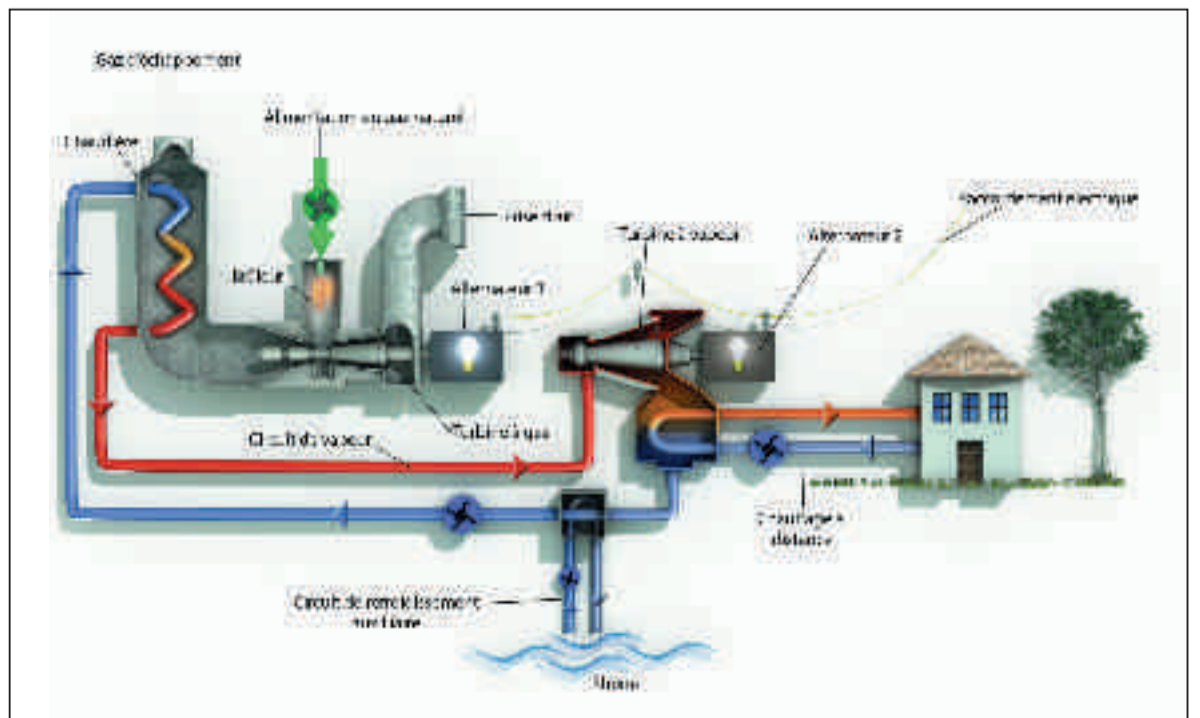
■ Fonctionnement d'une centrale thermique à gaz.
